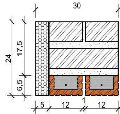
ЗОВНІШНЯ СТІНА
