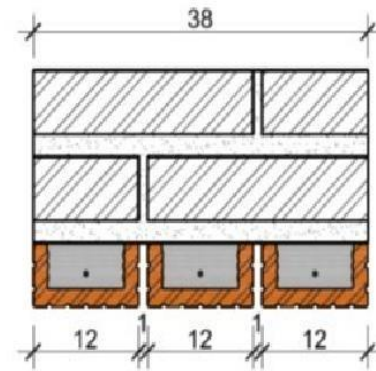
ВНУТРІШНЯ СТІНА
