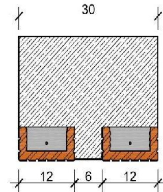
ВНУТРІШНЯ СТІНА
