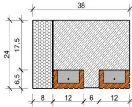
ЗОВНІШНЯ СТІНА
